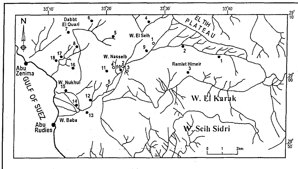
Fig.(2): Profiles (•) and water wells (°) location map of the studied plains and wadis. °1: Bir El Seih °2: Bir Nasseib °3: Bir Alluga °4: Bir Ramsa °5: Bir Rekas
